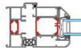
Jamb Detail
